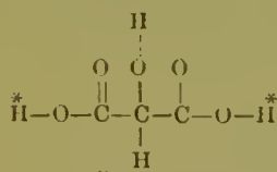
\text{C}_3\text{H}_2\text{O}_3(\text{OH})_2 Tartronsäure
